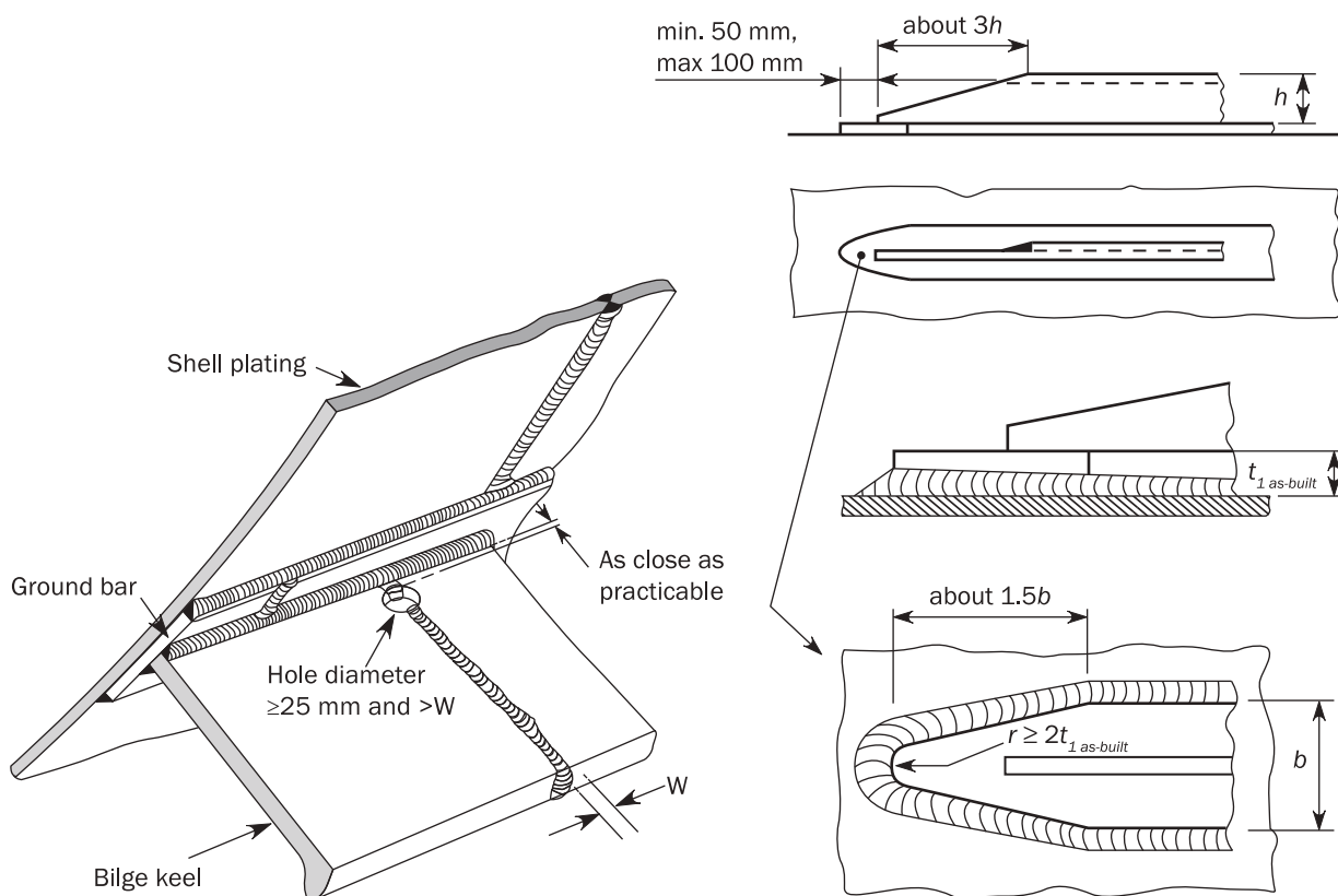
Figure 10 : Bilge keel
